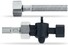
Aansluitslang DN 8 3/8" met 3/8" stopkraan
